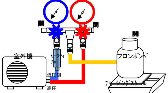
③ 冷媒充填
