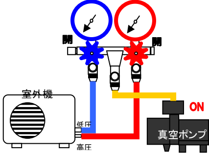
① 真空乾操作業
