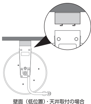
壁面（低位置）・天井取付の場合
