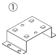
取付板 1個
