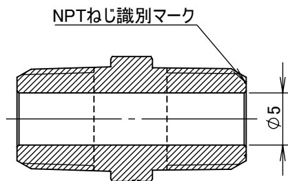
断面図 A-A
