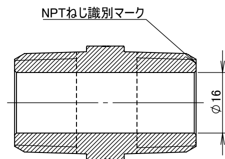
断面図 A-A
