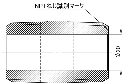
断面図 A-A
