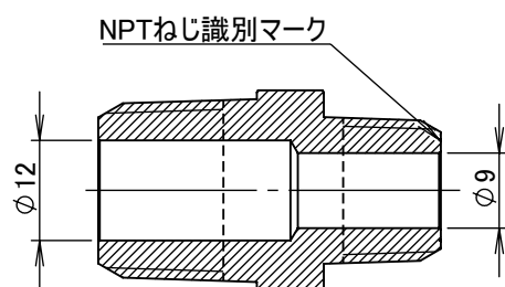
断面図 A-A
