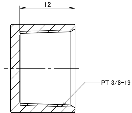
断面図 A-A
