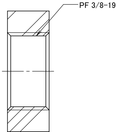
断面図 A-A
