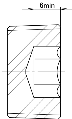
断面図 A-A
