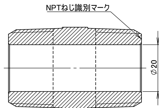
断面図 A-A
