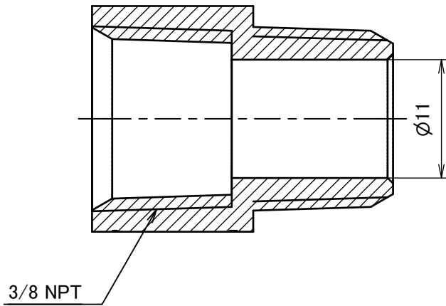
A-A (2:1)
