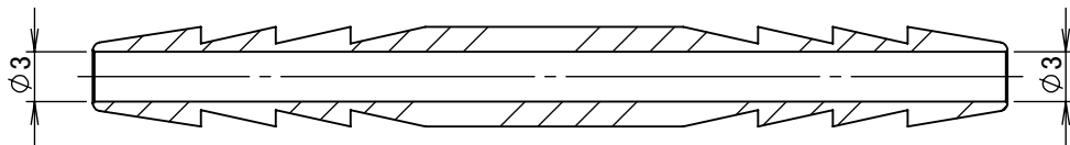
断面図 A-A
