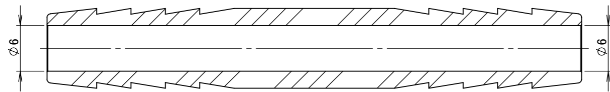
断面図 A-A
