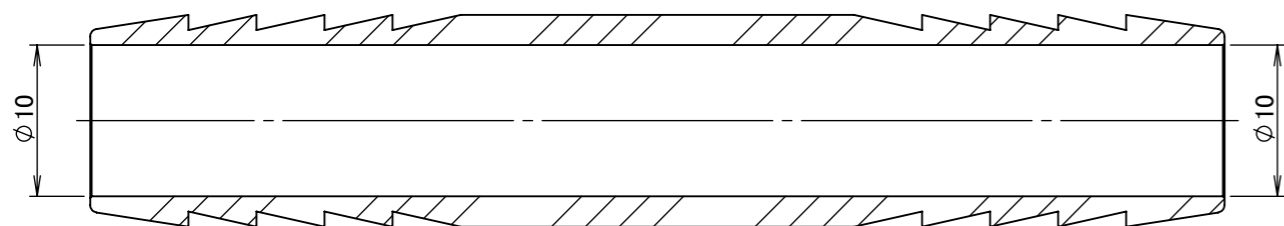
断面図 A-A
