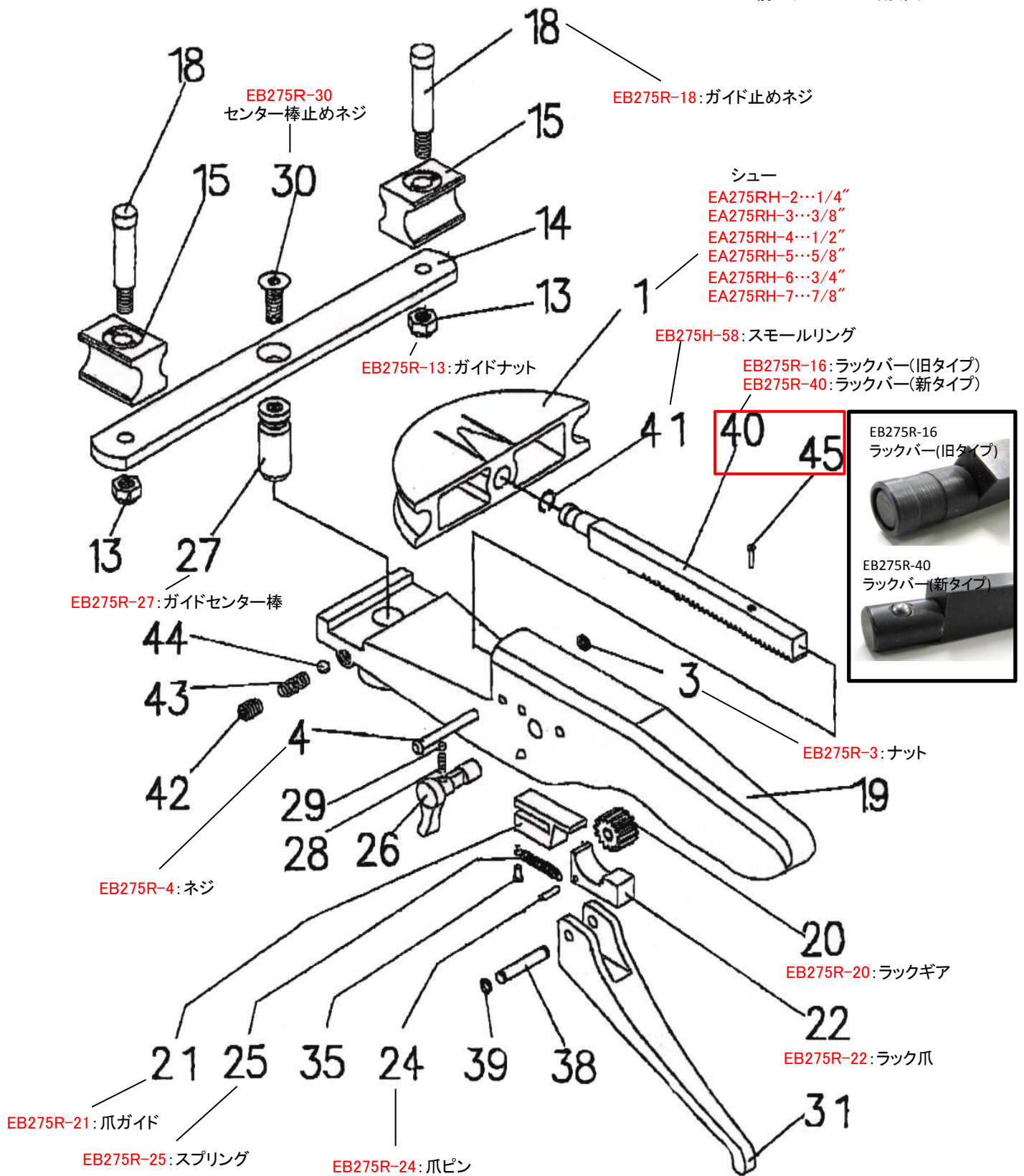
EB275H-45 <前モデル>シュー用蝶ネジ
