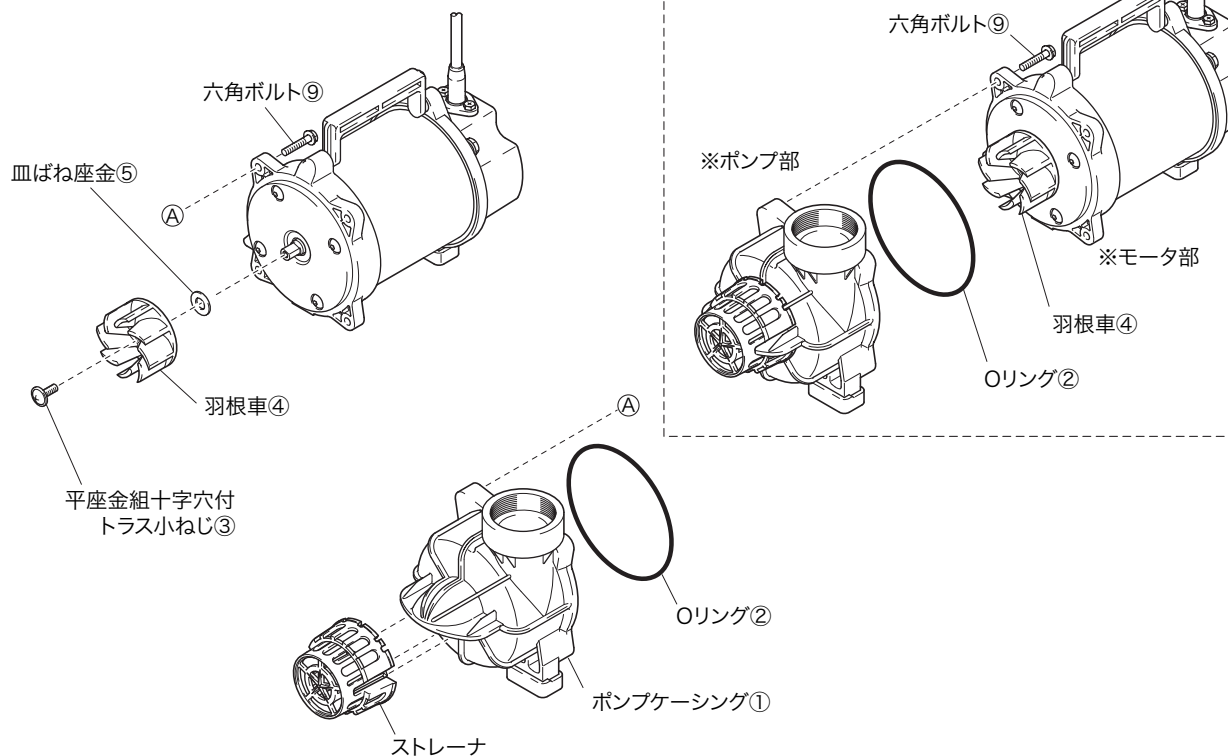
〔ポンプ部分解図〕
