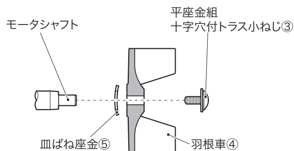
[皿ばね座金の組み付け方向]
