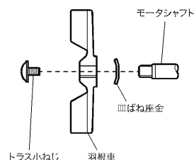
【皿ばね座金の組付け方向】
