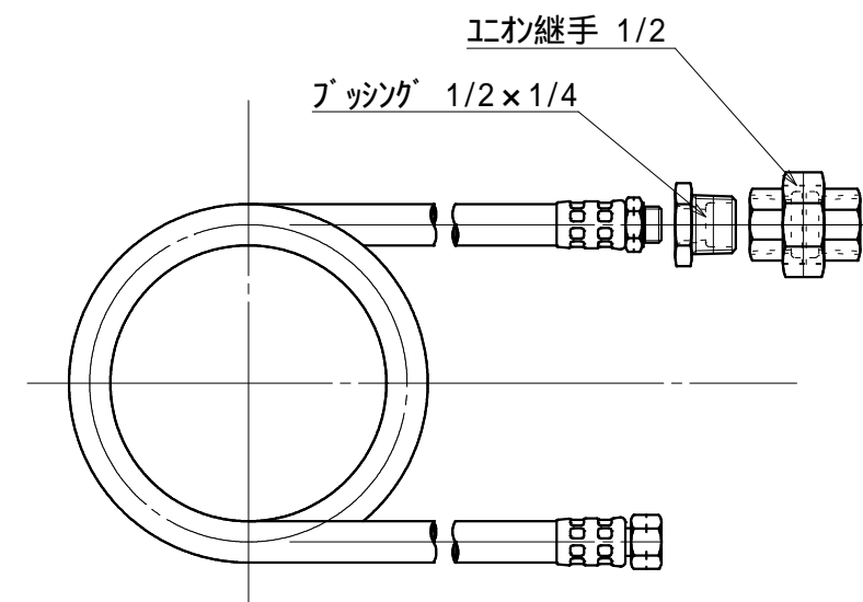
付属ホース
