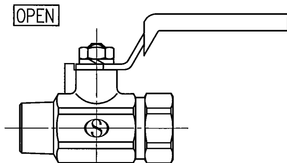
外觀図
