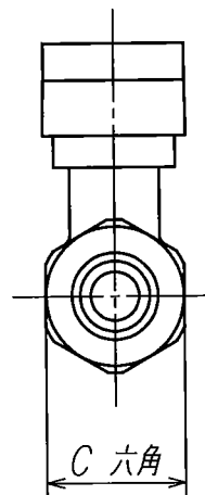
外観図
