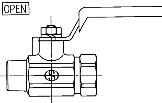
外観図
