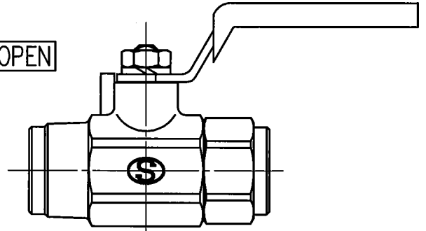
外観図
