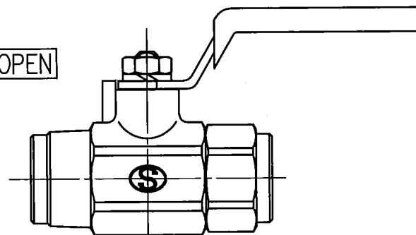
外觀図
