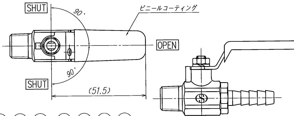
外観図
