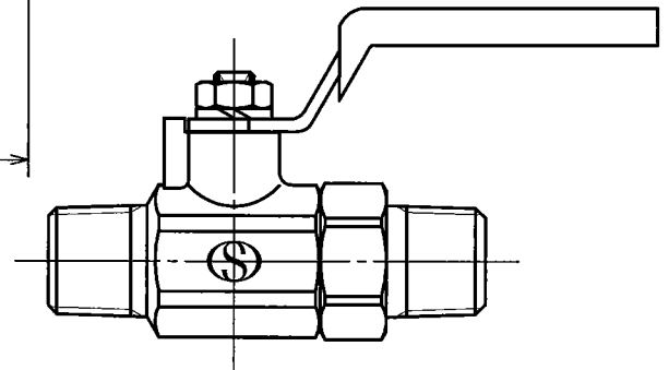
外觀図
