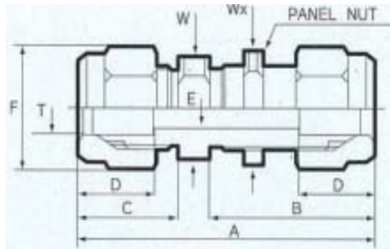
図面のWは四角対辺の寸法です。
