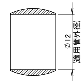
断面図 A-A
