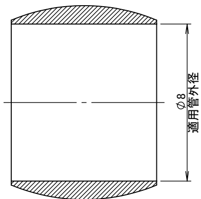
断面図 A-A
