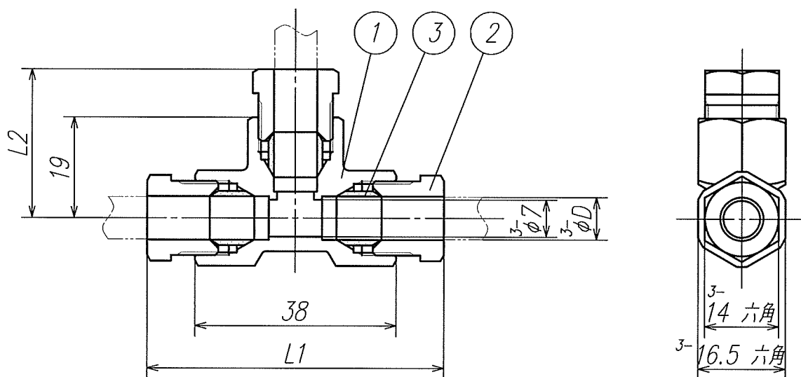
外觀図
