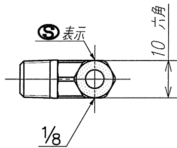
A-A'断面
