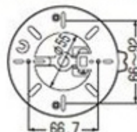
■共通フランジ寸法
