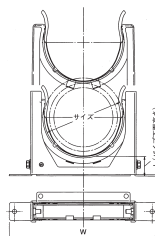
耐火二層管用 (TVP仕様) 40A~65A ※75A~100Aは形状が変わります。
