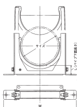
VU管 50A~100A VP管用 40A~100A
