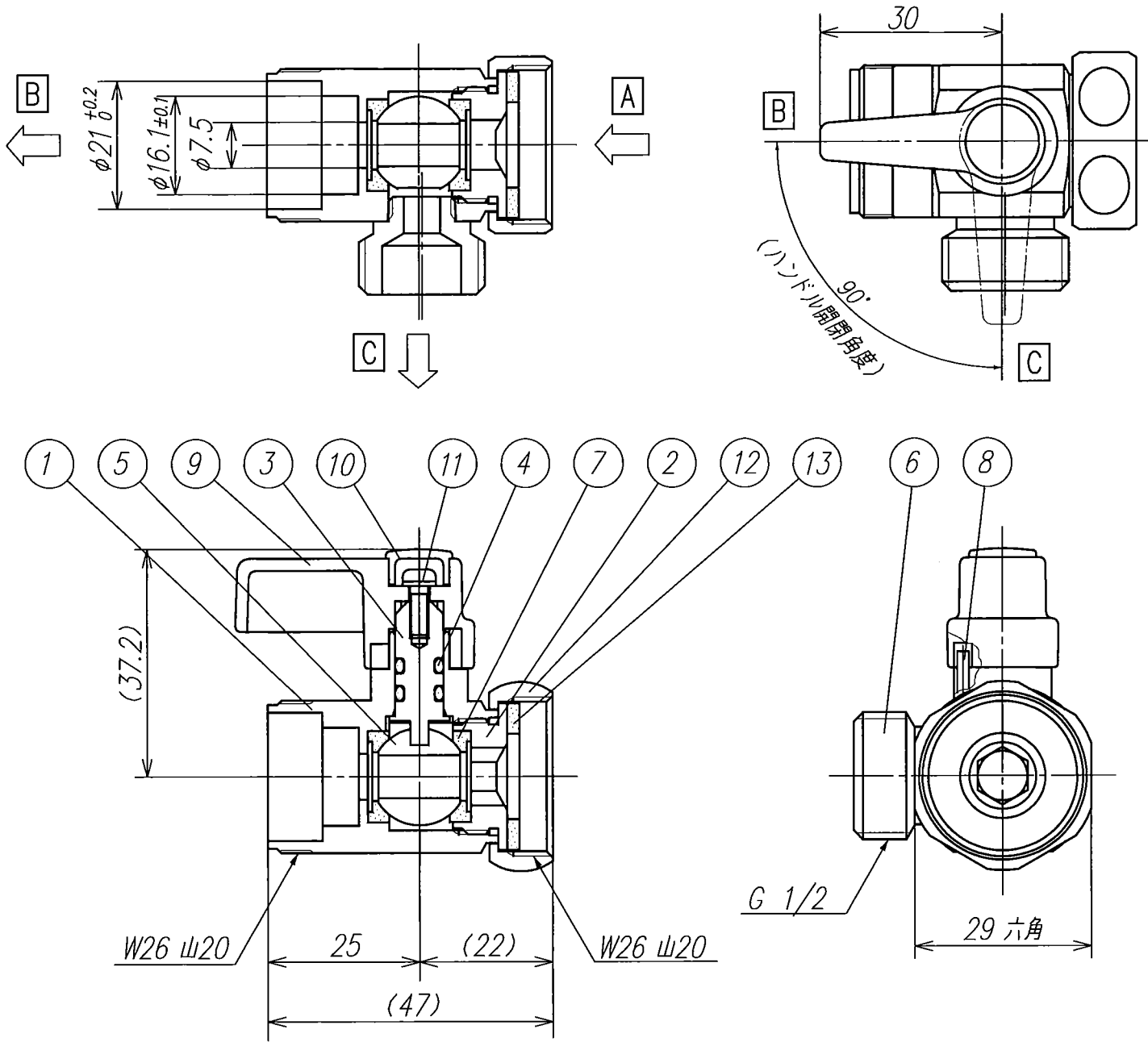
2) 本図の状態より、ハンドル反時計回り90°回転にて、AC間OPEN、B側SHUTとなる 注記 1) 本図は、AB間OPEN、C側SHUT状態である
