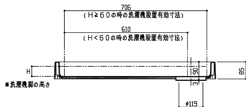
断面A-A
