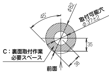
図1. 裏面取付作業必要スペース寸法(1:5)
