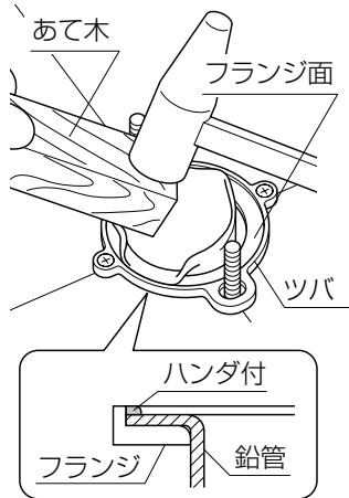
仕上げ後のフランジ断面
