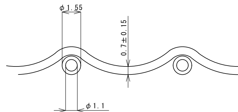
断面詳細
