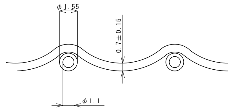
断面詳細
