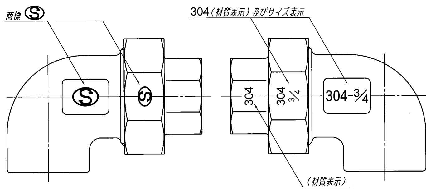
外觀図
