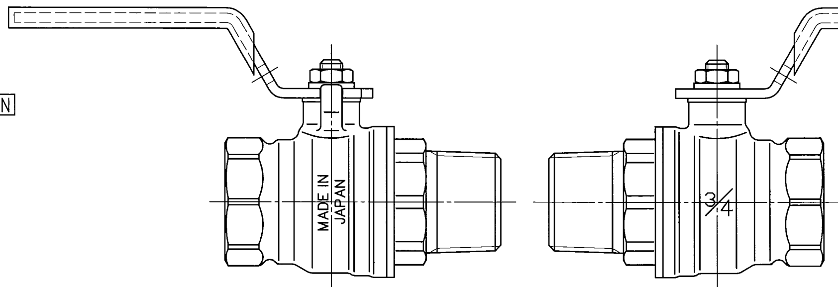
外観図
