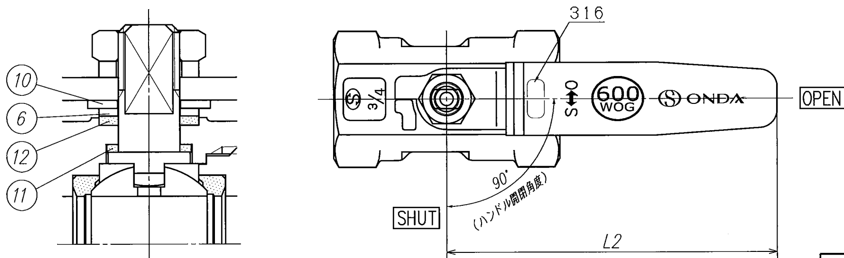
C部詳細
