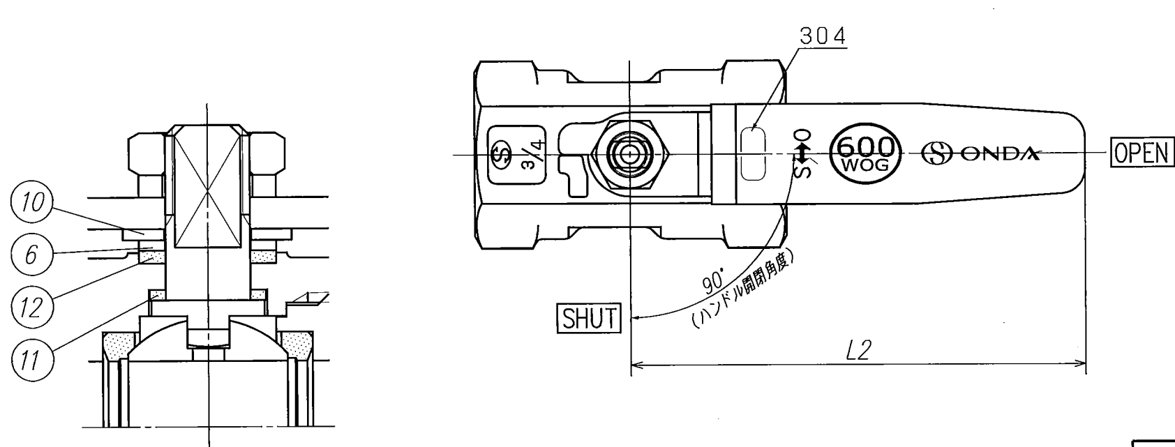
C部詳細
