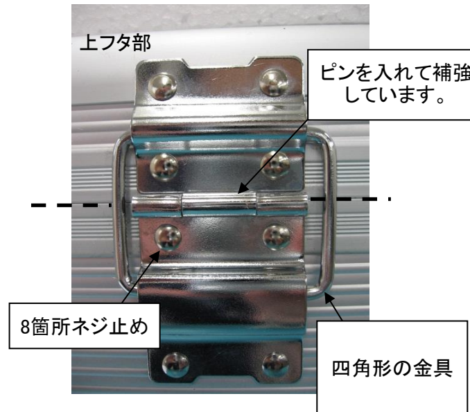
ケース裏の丁番の仕組み
