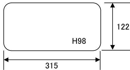
本体内寸法(単位:mm)
