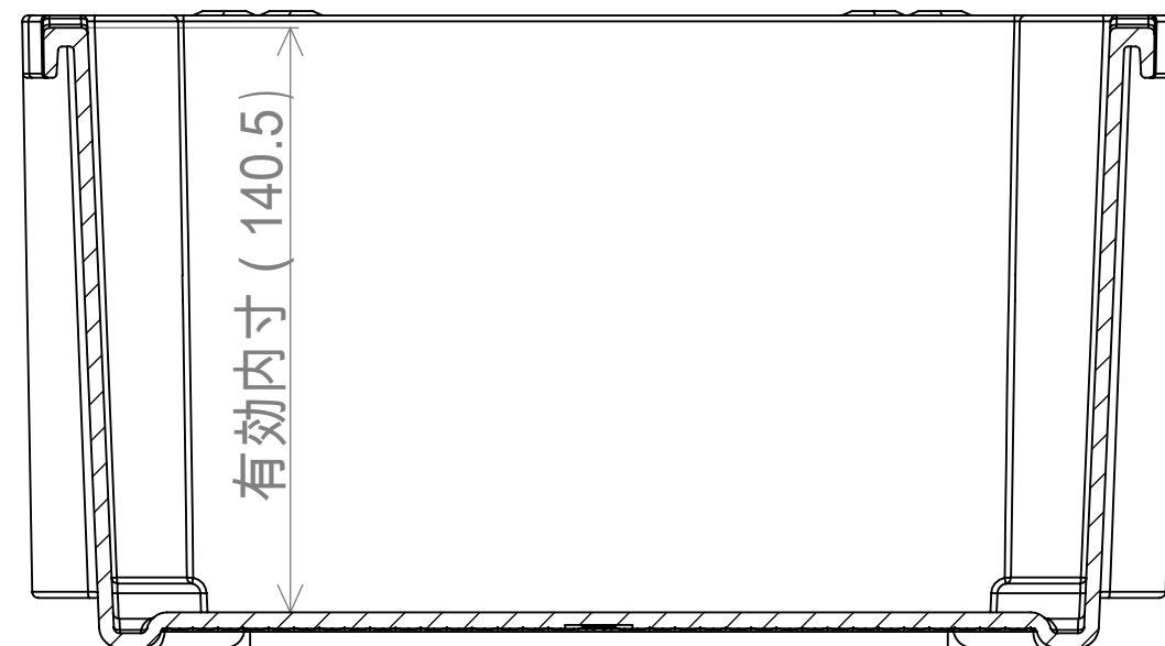
断面图 A-A
