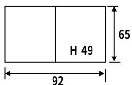
内寸法
