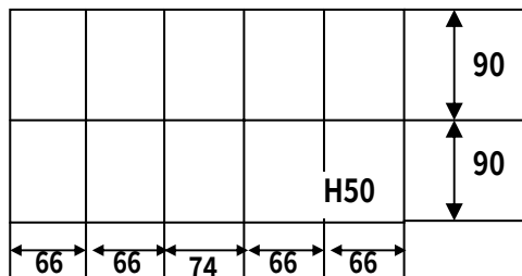
中皿内寸法
