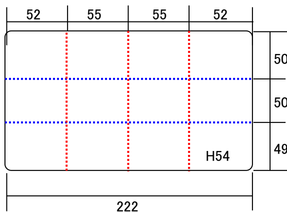
本体内寸法
