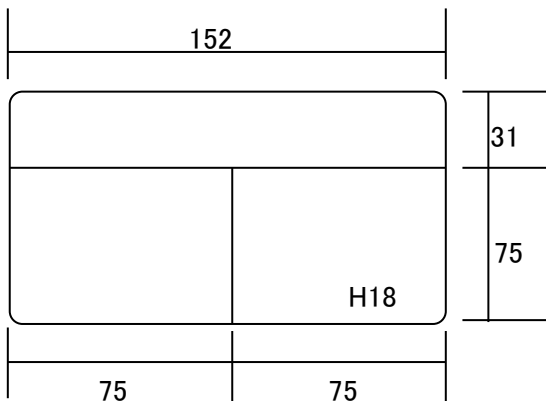
中皿寸法
