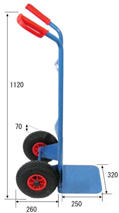
・全体図(2) (単位:mm)
