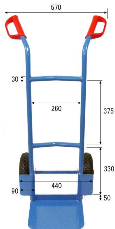
・全体図(1) (単位:mm)
