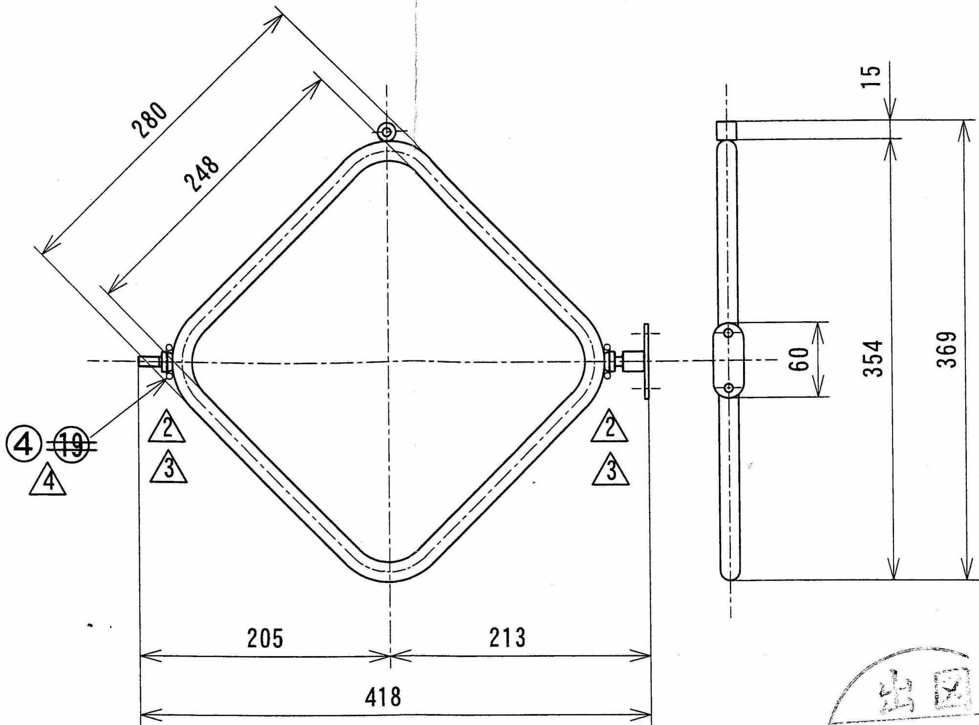
一斗缶ホルダー形状
