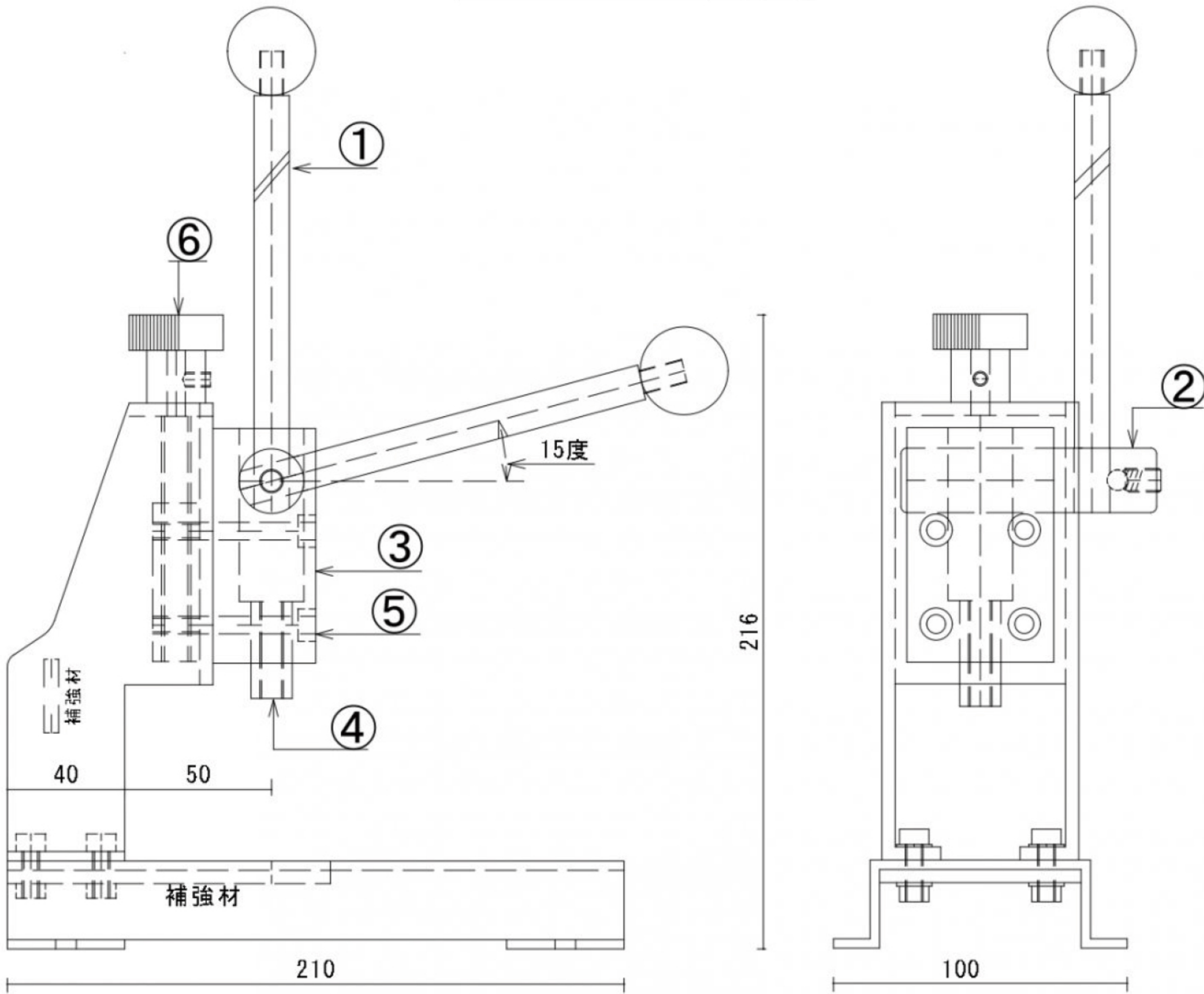
CSP-11S寸法図
